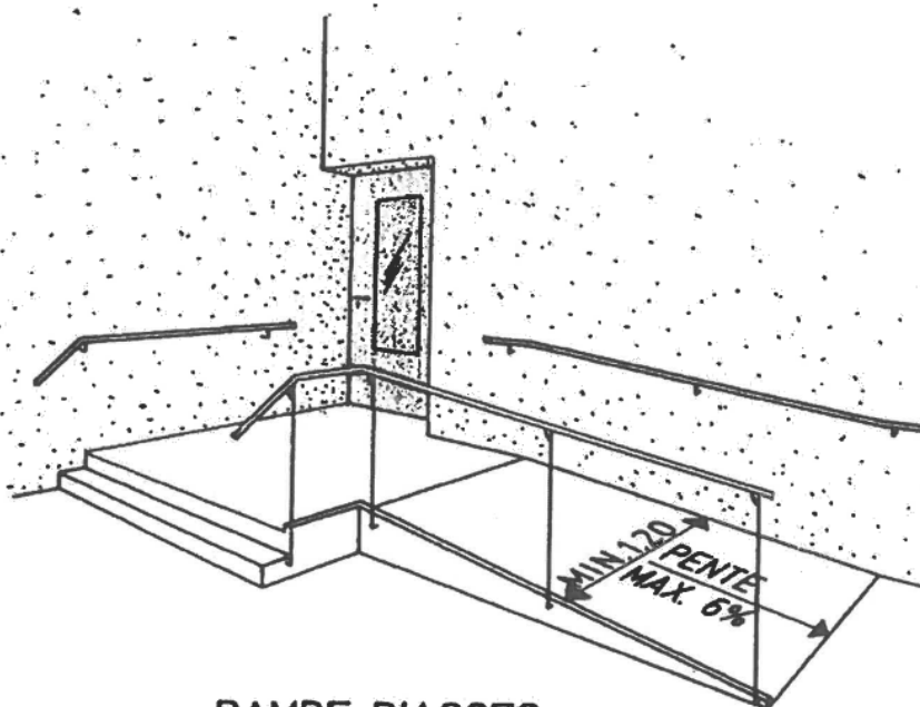
RAMPE D'ACCES
